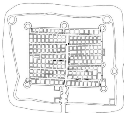
شکل (۹) نقشه وضع موجود قلعه سریزد (مأخذ: آرشیو پایگاه میراث فرهنگی شهر تاریخی مهریز)
